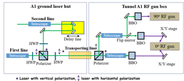
Figure 2: トランスポートライン
