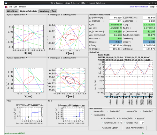
Figure 10: 5sector ワイヤースキャナー
