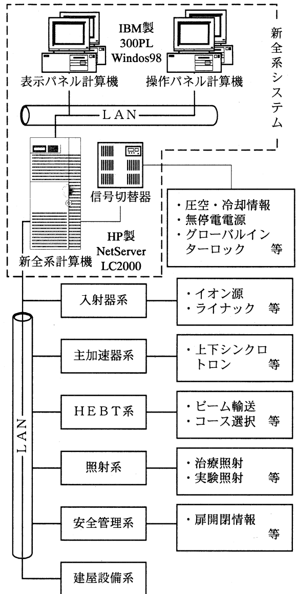
図 2. システム構成
