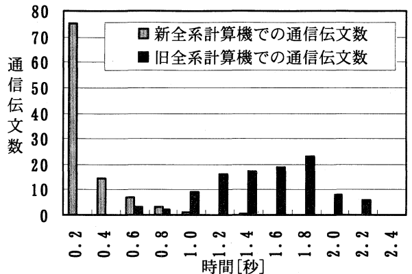
図5. 新旧全系計算機での受信から送信までに要した処理時間と通信伝文数
